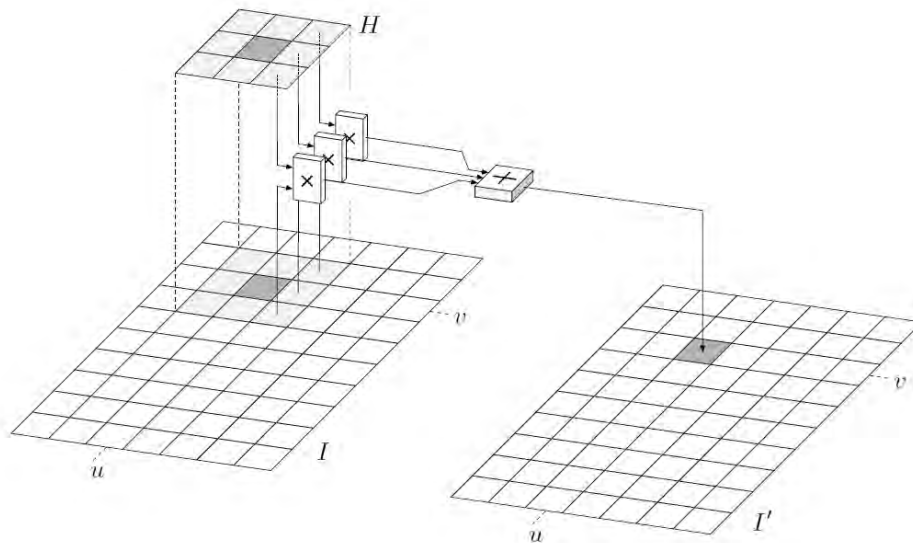
Abbildung 4.2: Anwendung eines linearen Filters . An jeder Position (u, v) im Bild wird die Filtermatrix so positioniert, dass der Hot Spot auf die aktuelle Position fällt. Anschließend werden alle Bildpunkte mit den darüber liegenden Koeffizienten multipliziert. Die Ergebnisse werden jeweils aufsummiert und am Ende als Ergebnis-Wert an der aktuellen Position (u, v) gespeichert (entnommen aus (author?) [22]).
