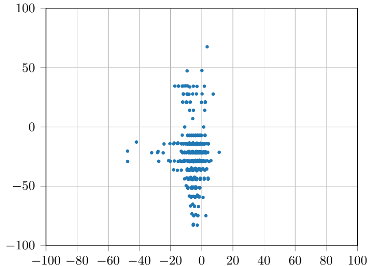
Abbildung 6.6: Die Abbildung zeigt den Fehler der Vorhersagen des B-Human -Detektors (in blau) in Relation zur tatsächlichen Position des Roboters an Koordinate (0, 0) . Einheiten in Millimeter.
