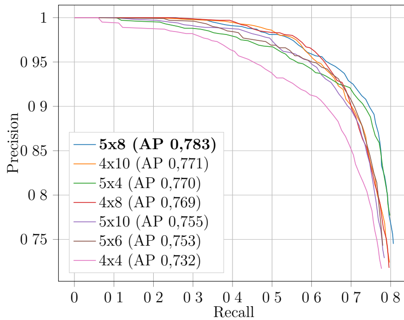
Abbildung 5.11: Precision-Recall-Kurve verschiedener Modelle. Die x -Achse beschreibt den Recall – die y -Achse die Precision . Der Legende sind die getesteten Größen ( M \times N ) und die Average Precision ( AP ) zu entnehmen.
