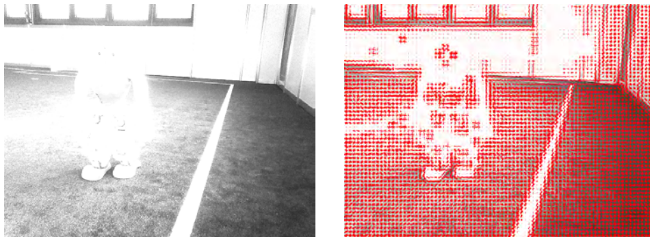
Abbildung 6.5: Die Abbildung zeigt ein stark überbelichtetes Bild (links) und einen zugehörigen HoG -Deskriptor (rechts). Die Normalisierung in den HoG -Deskriptoren sorgt dafür, dass einige Gradienten trotz starker Überbelichtung erhalten bleiben. Trotzdem fehlen insbesondere viele Details. Einige Teile, wie die Arme oder der Kopf, sind außerdem nicht vollständig. Die Kombination von fehlenden Teilen und Details sorgt dafür, dass die Detektion fehlschlägt.
