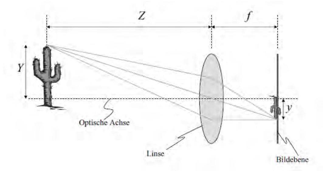
Abbildung 4.9: Darstellung der “dünnen Linse”. Das entstehende Modell ist dem Lochkamera-Modell sehr ähnlich. Die Linse wird dabei als symmetrisch und unendlich dünn angenommen. Lichtstrahlen werden an einer virtuellen Ebene in der Linsenmitte gebrochen, wobei sich die gleiche Abbildungsgeometrie wie bei der Lochkamera ergibt (entnommen aus [22, Seite 9]).
