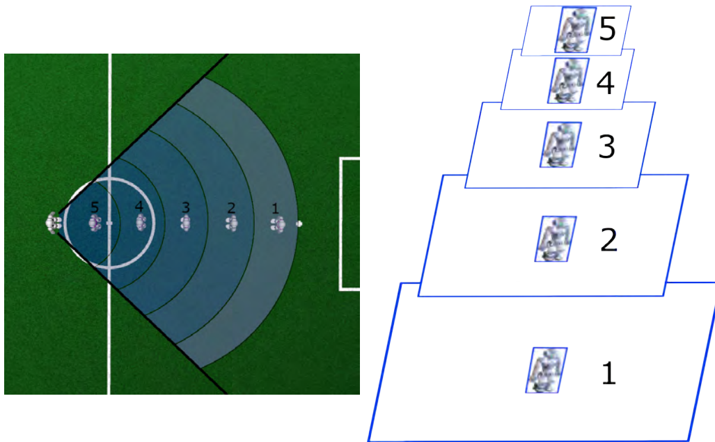
Abbildung 5.3: Beispiel-Zeichnung für 5 Level . In der linken Abbildung begrenzen die schwarzen Linien den Sichtbereich des Roboters. Die Level sind in verschiedenen Blautönen eingefärbt und durchnummeriert dargestellt. Level 1 beschreibt hier das erste Level einer Merkmal-Pyramide und somit das voll aufgelöste Bild. Je weiter man nun die Pyramide durchläuft, desto kleiner wird das verarbeitete Bild und somit auch der Abdeckungs-Bereich der Teil-Filter – wie auch in der rechten Abbildung zu sehen ist. Die Übergänge zwischen den einzelnen Bereichen sind fließend. Das heißt, dass mehrere Level für den selben Roboter hohe Bewertungen erreichen können. Befinden sich einer oder mehrere der Bereiche außerhalb des Spielfeldes, werden sie nicht berücksichtigt.
