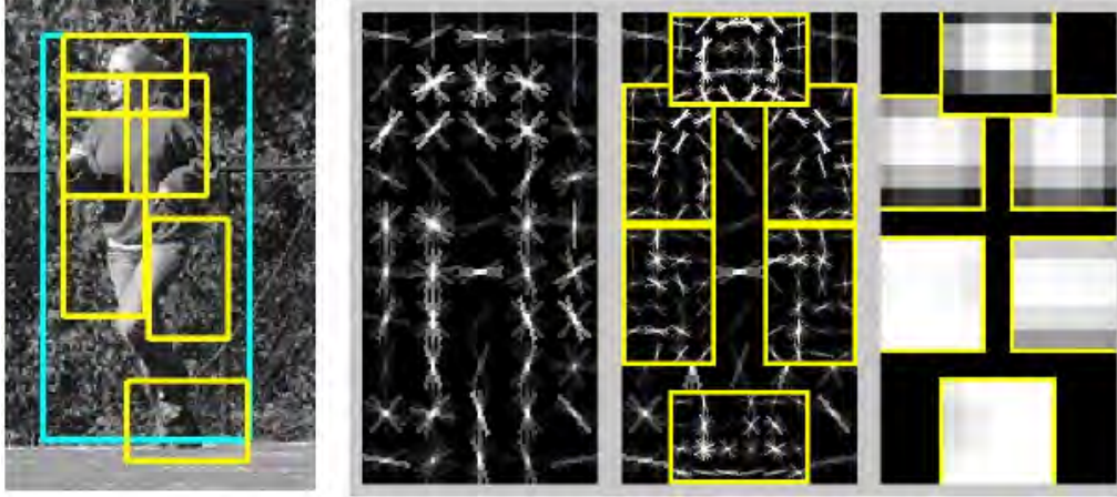
Abbildung 4.6: Beispiel für ein Deformable Part Model . Das Modell wird definiert durch eine Wurzel (2. von links) und mehreren höher aufgelösten Teilen (2. von rechts). Auf der rechten Seite sind die deformation costs abgebildet. Links ist eine beispielhafte Detektion einer Person zu sehen. Die Wurzel wird in blau dargestellt, die anderen Teile in gelb (entnommen aus [1]).
