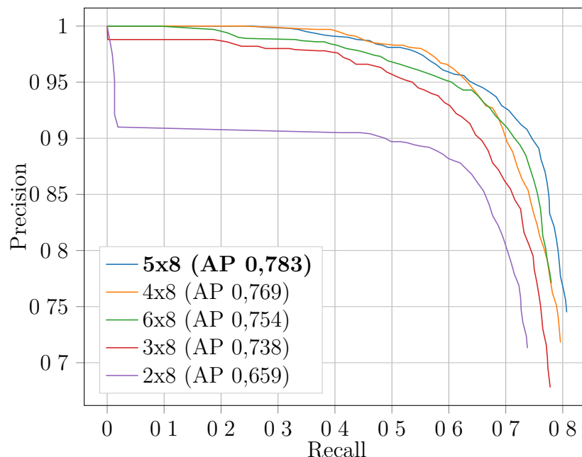
Abbildung 5.10: Precision-Recall-Kurve verschiedener Modelle. Die x -Achse beschreibt den Recall – die y -Achse die Precision . Der Legende sind die getesteten Größen ( M \times N ) und die Average Precision ( AP ) zu entnehmen. Die Modelle wurden bis zu einer Größe von 5 \times 8 immer besser, ehe die Ergebnisse mit einem Modell von einer Größe von 6 \times 8 wieder deutlich schlechter wurden.
