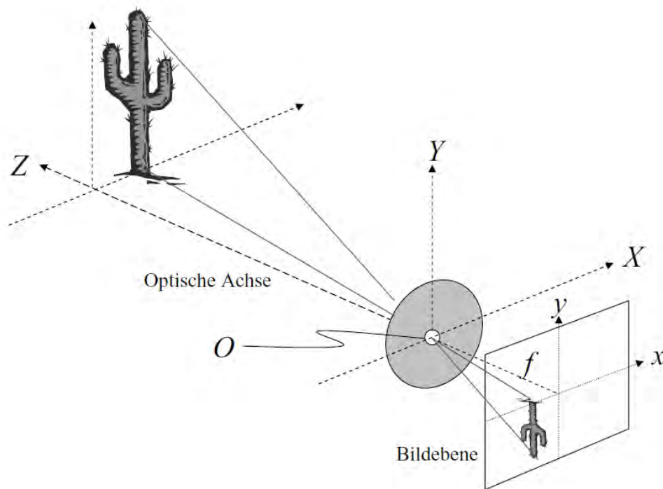
Abbildung 4.8: Darstellung des Lochkamera-Modells. Bei diesem Modell besteht die Kamera aus einer geschlossenen Box mit einer sehr kleinen Öffnung an der Vorderseite. Die Bildebene befindet sich an der gegenüberliegenden Seite. Lichtstrahlen, die durch die Öffnung fallen, werden geradlinig an die Bildebene projiziert, womit ein verkleinertes, horizontal gespiegeltes Abbild an der Bildebene entsteht (entnommen aus [22, Seite 7]).
