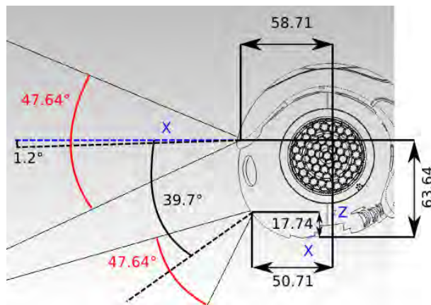
(b) Positionierung und Ausrichtung der beiden Kameras des NAO Roboters (entnommen aus [19]).
