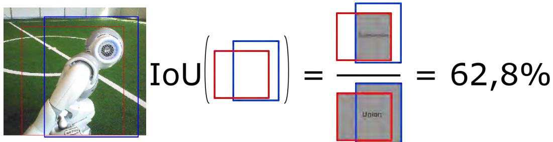
Abbildung 4.10: Beispiel für eine IoU -Berechnung. Die ground-truth Bounding-Box wird in rot dargestellt, die Detektion des Roboters in blau. Die für die Berechnung relevanten Flächen sind grau markiert.
