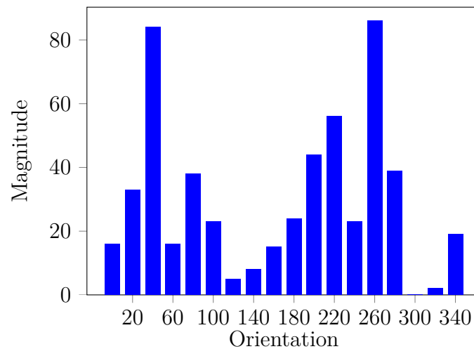
Abbildung 4.5: Histogramm der hervorgehobenen Zelle aus Abbildung 4.4. Die x -Achse zeigt die Einträge, welche die Orientations von 0 bis 360 Grad gleichmäßig unterteilen. Eine Orientation von 0 und eine von 360 Grad werden hier als gleich angesehen. Die y -Achse zeigt die aufsummierten Magnitudes . Dieses Histogramm repräsentiert einen (unnormalisierten) HoG -Deskriptor.
