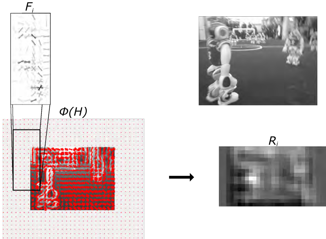
Abbildung 5.6: Beispiel für die Berechnung von Filter -Antworten. Der Filter F_i wird wie bei einer Faltung über die Merkmals-Vektoren \phi(H) geschoben. Der Hot Spot befindet sich dabei in der linken oberen Ecke des Filters . Da der vordere Roboter in diesem Bild sehr groß ist, ergeben sich erst auf höheren Leveln hohe Filter -Antworten. Tiefe Filter -Antworten sind in schwarz dargestellt – hohe in weiß. In den Antworten auf der rechten Seite sieht man deutlich, wie die Werte an der Position des vorderen Roboters ausschlagen.
