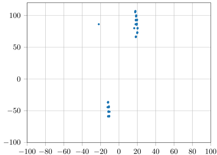
Abbildung 6.7: Die Abbildung zeigt den Fehler der Vorhersagen des Hybrid-Modells (in blau) in Relation zur tatsächlichen Position des Roboters an Koordinate (0,0) . Einheiten in Millimeter.
