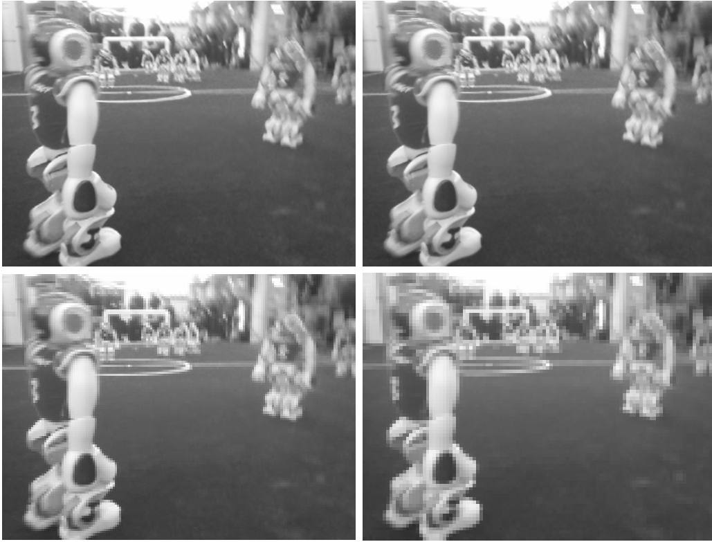
Abbildung 5.5: Verschieden skalierte Versionen eines Eingabebildes. Selbst bei sehr kleinen Skalierungen gehen nur wenige Gradienten verloren. Die Skalierungen (Vielfache der Original-Auflösung) von links oben nach rechts unten: 1, 0,57, 0,25, 0,16.
