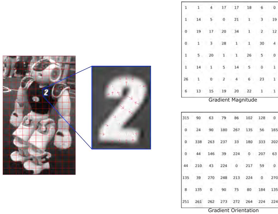
Abbildung 4.4: Die Abbildung zeigt ein Beispiel für die Magnitudes und Orientations in einer Zelle. Auf der linken Seite ist zu sehen, wie das Eingabebild in Zellen unterteilt wird (in rot dargestellt). In der Mitte sieht man die Orientations (rot) einer bestimmten Zelle skaliert nach der Magnitude . Auf der rechten Seite sind die Magnitudes (oben) und die Orientations (unten) der Zelle dargestellt. Aus diesen Zellen werden anhand der Magnitude und Orientation Histogramme mit 18 Einträgen berechnet. In diesen Einträgen werden die Magnitudes interpoliert und auf Basis ihrer Orientation aufsummiert.
