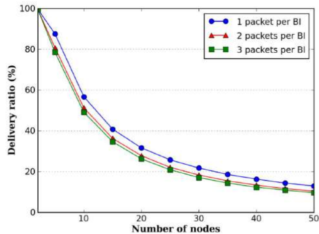
ABBILDUNG 3.6: Einfluss der Paketrage auf die Zuverlässigkeit des klassischen 802.15.4 MAC Layers ([ACF11, vgl. S. 11])
